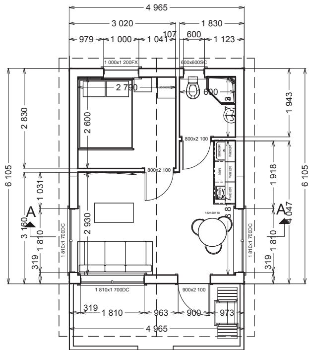
GRUNNMYND 1:50
