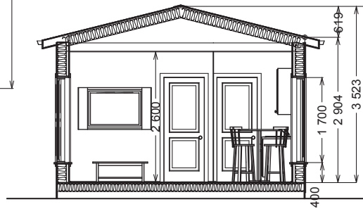
SKURÐUR A, 1:50
