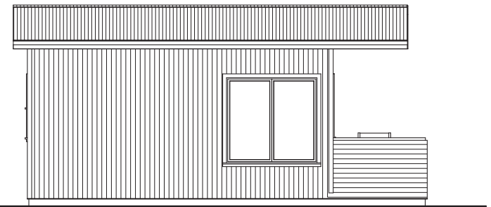
VINSTRI HLIÐ, 1:50
