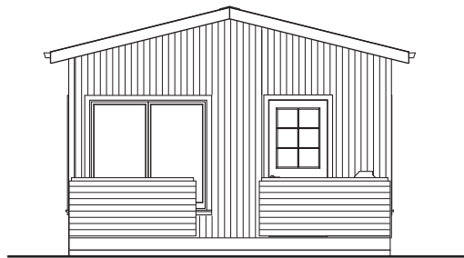
FRAMHLIÐ, 1:50
