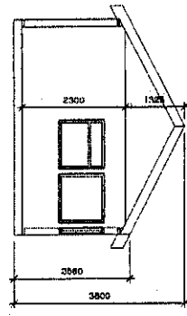
A 1:50
