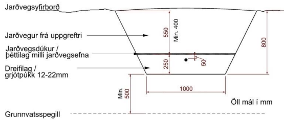
Mynd 12. Dæmi um hreinsiskurð – snið.
