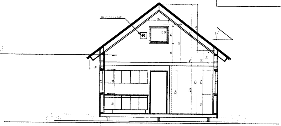
SNID A-A 1:50
