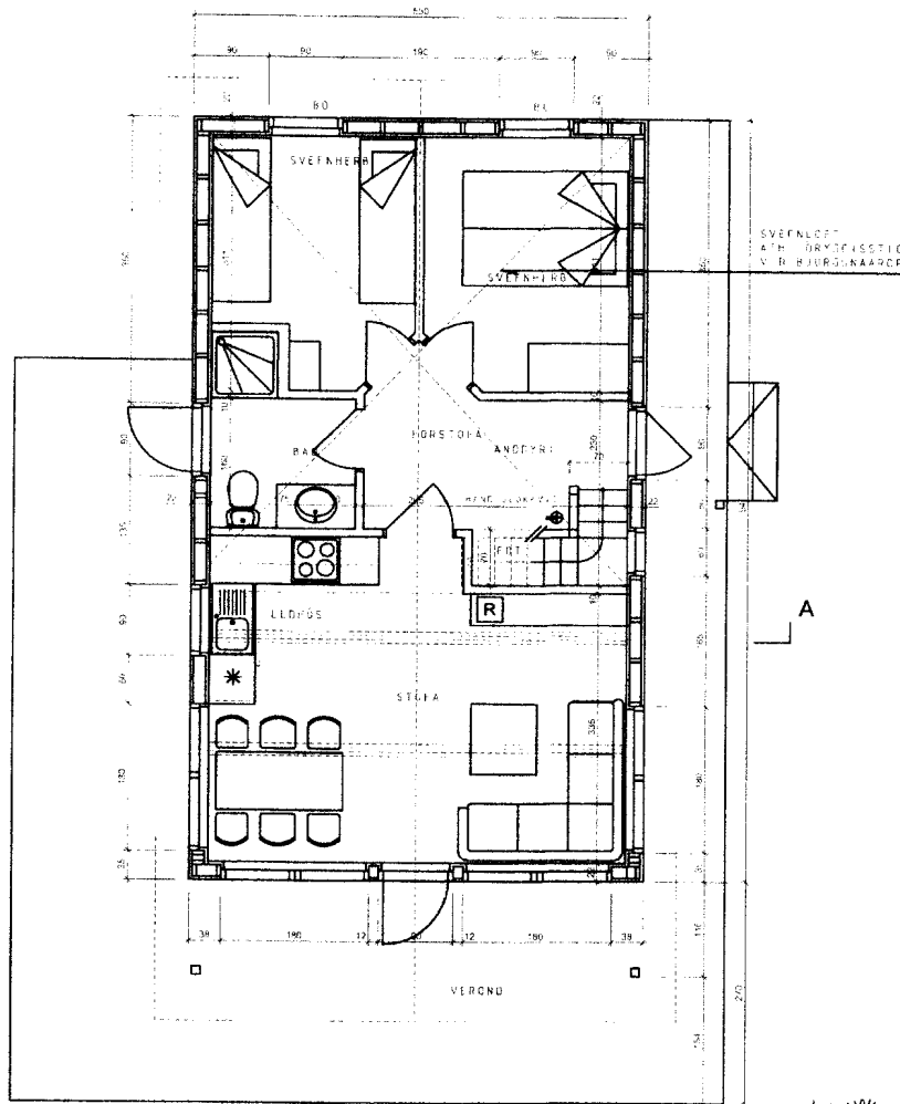
GRUNNMYND 1:50
