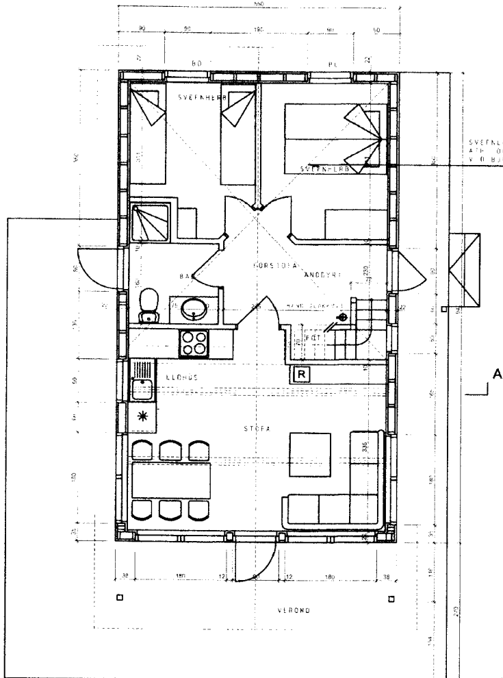
GRUNNMYND 1:50
